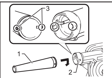
► 1. Boquilla 2. Toma del soplador 3. Clavija o protuberancia
